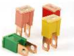
5.41 Serie 294 Innesto Maschio
